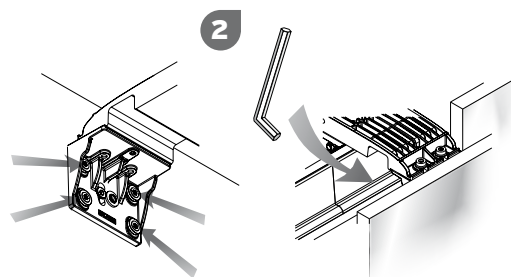
Fori di collegamento alla struttura Trous de connection à la structure Connecting holes to the structure Bohrungen für die Verbindung der Struktur
