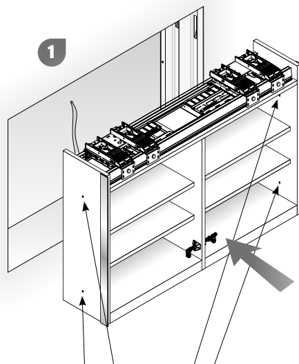
Fori di collegamento alla struttura Trous de connection à la structure Connecting holes to the structure Bohrungen für die Verbindung der Struktur
